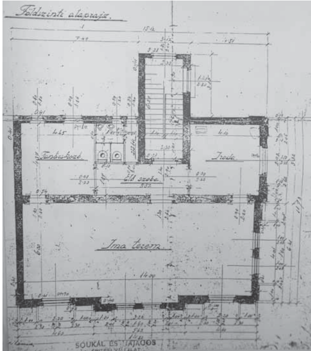
A tervezett Imaház földszinti alaprajza
