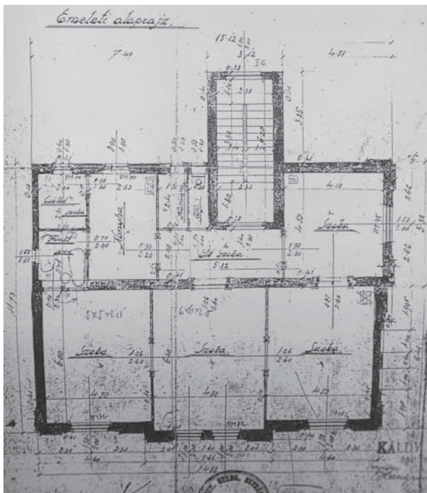
A tervezett Imaház emeleti alaprajza
